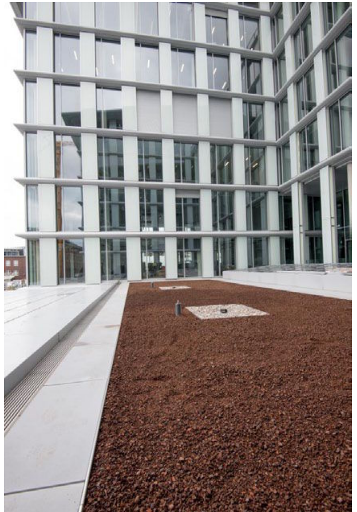
Auf die verschweißte Abdichtungsbahn und die direkt darunterliegenden Dämmelemente aus Neopor® wurden Boden für die Begrünung und teilweise auch Gehwegplatten aufgebracht.
